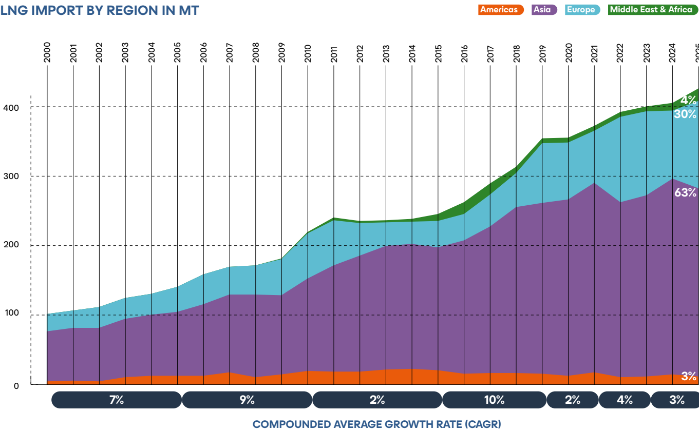
LNG IMPORT BY REGION IN MT
