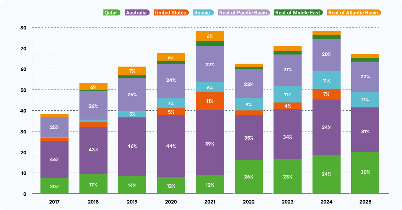
CHINA LNG BY SOURCE (MT)
